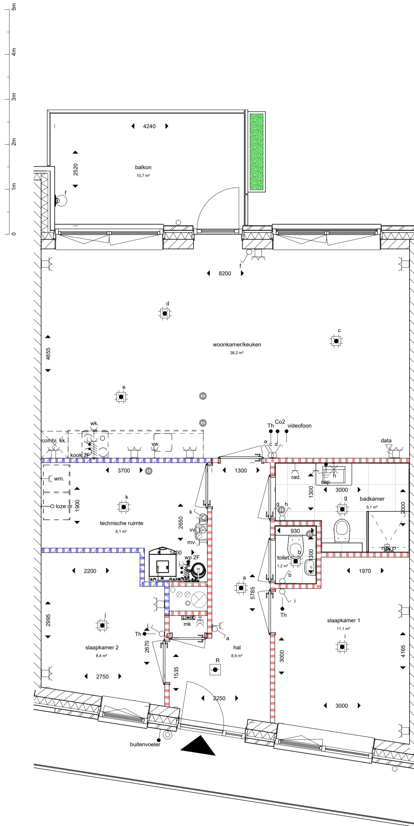
bnr 20 - type (Jardin du Luxembourg)
