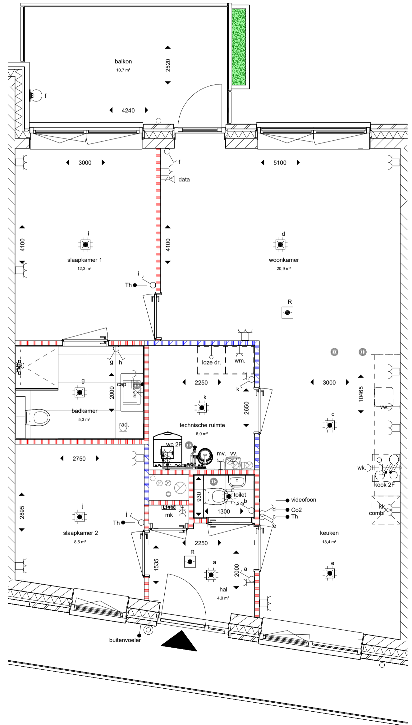
bnr 09 - type (Hyde Park) 1 : 50
