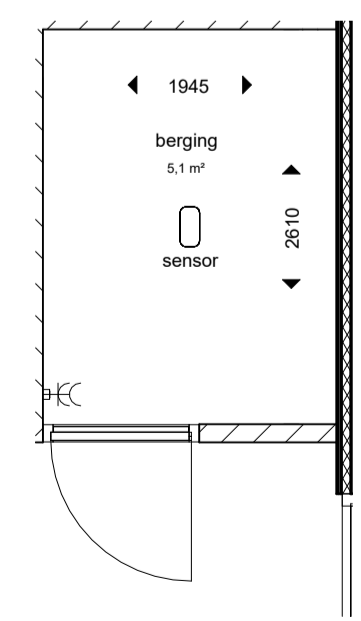
berging 1 : 50 De genoemde maten zijn circa maten, aangeduid in millimeters.
