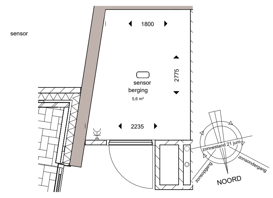
berging 1 : 50 De genoemde maten zijn circa maten, aangeduid in millimeters.
