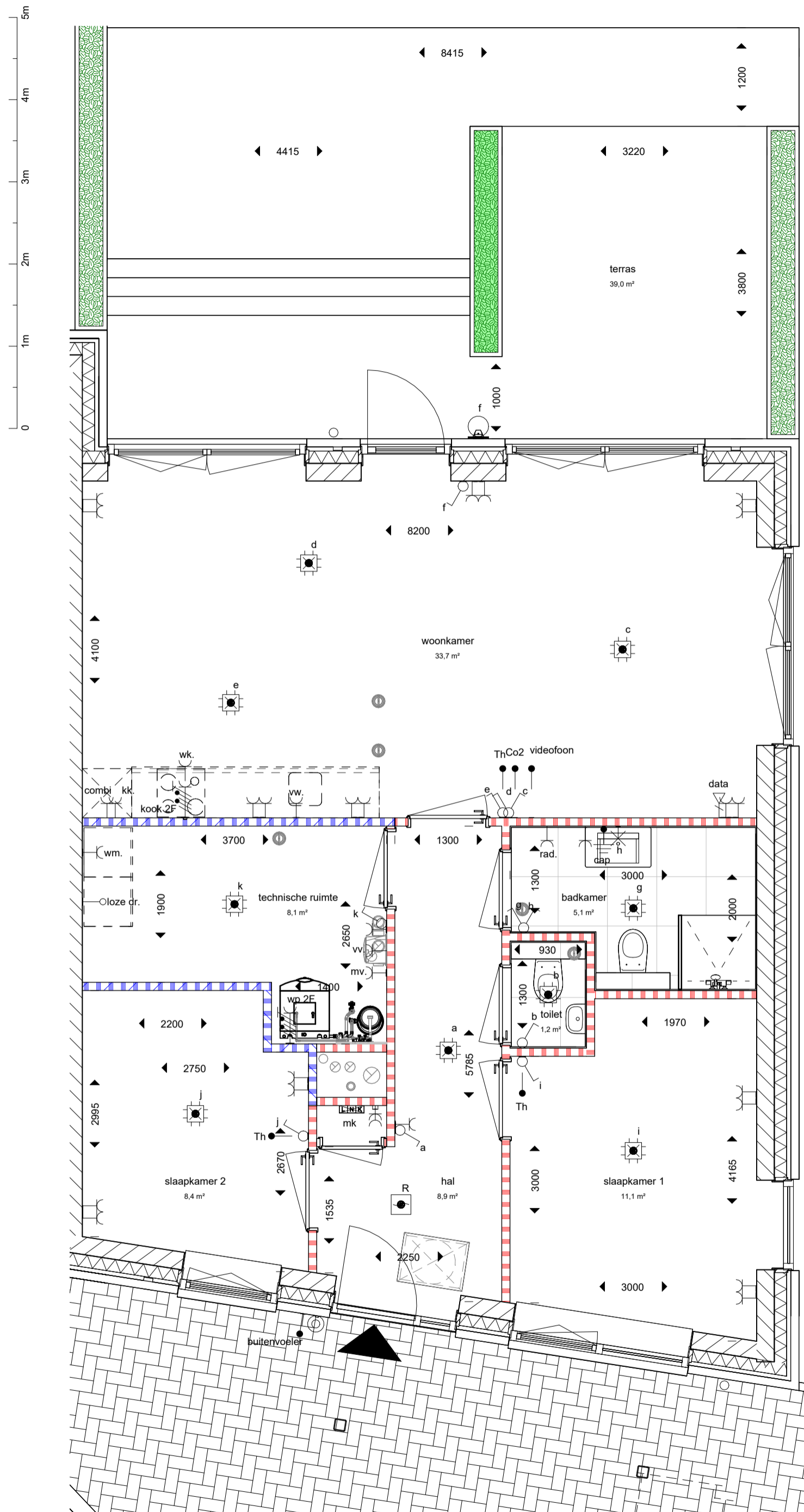
bnr 01 - type (Zuiderpark)
