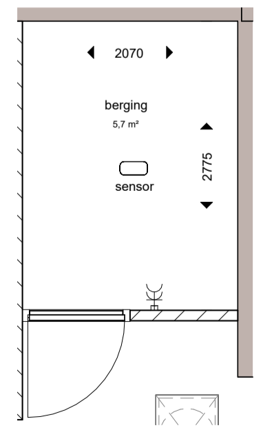
berging 1 : 50
