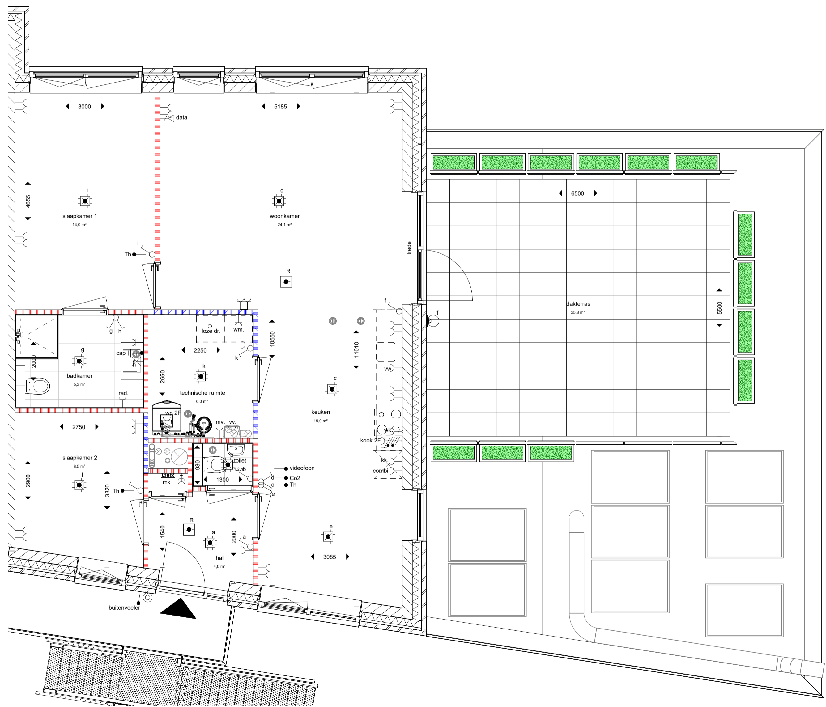
bnr 45 - type (Central Park) 1 : 50
