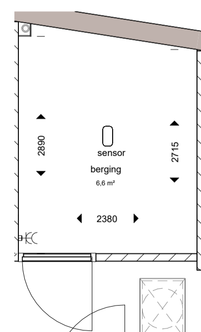
berging 1 : 50
