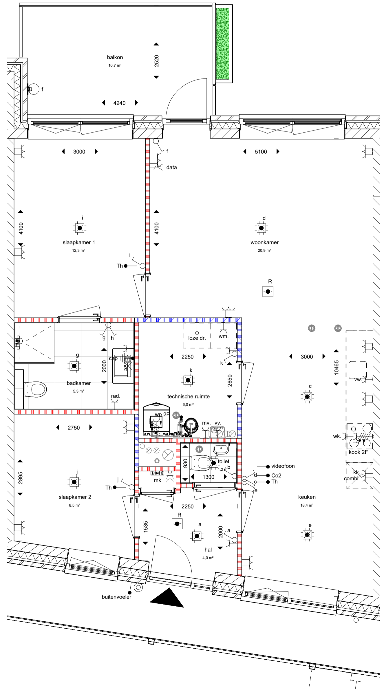
bnr 24 - type (Hyde Park) 1 : 50
