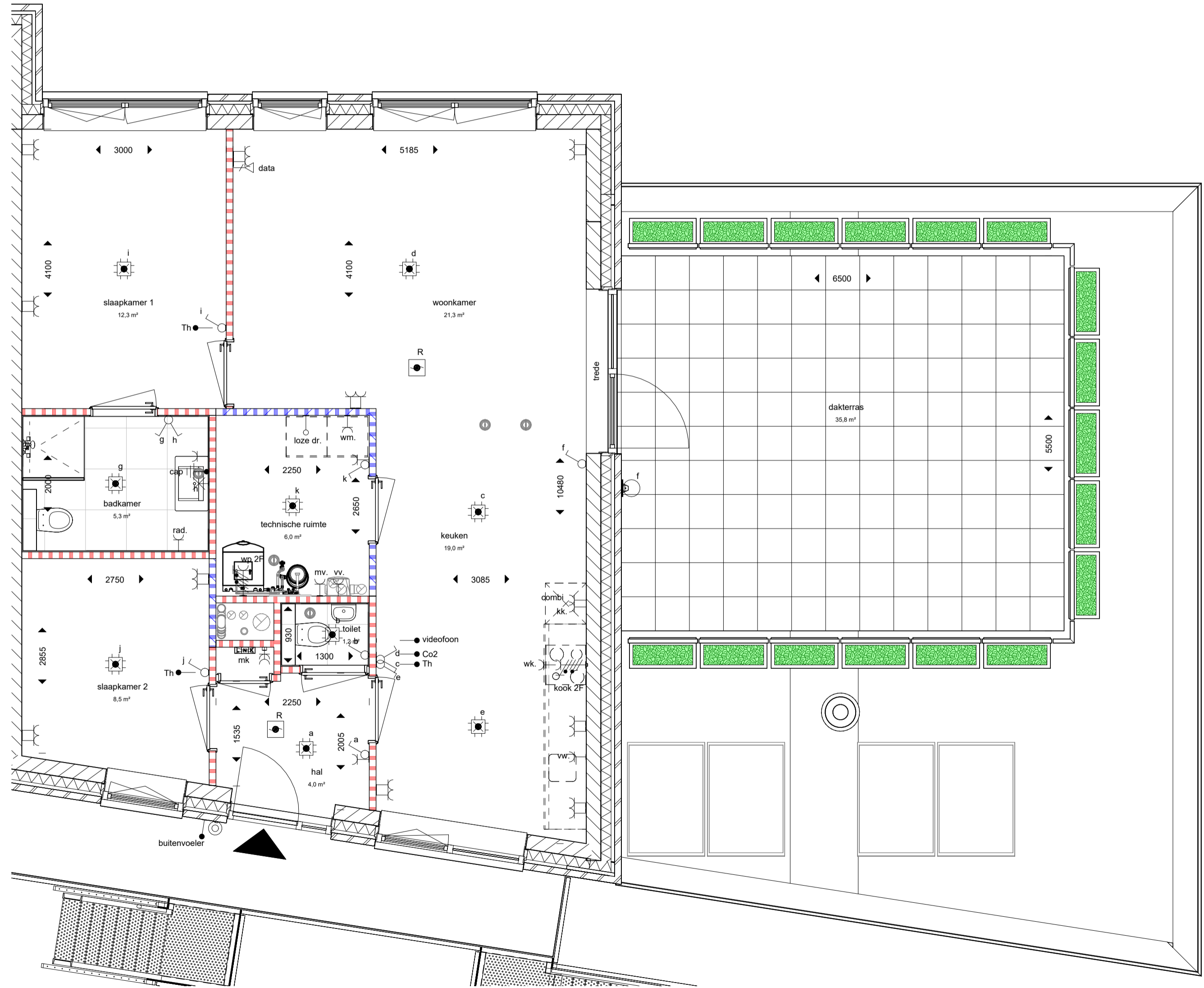
bnr 30 - type (Hyde Park) 1 : 50
