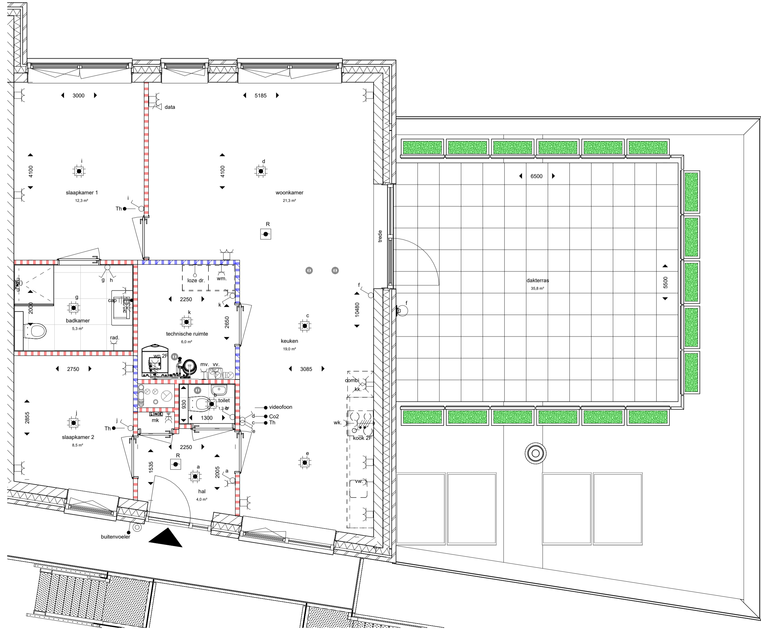
bnr 15 - type (Hyde Park) 1 : 50
