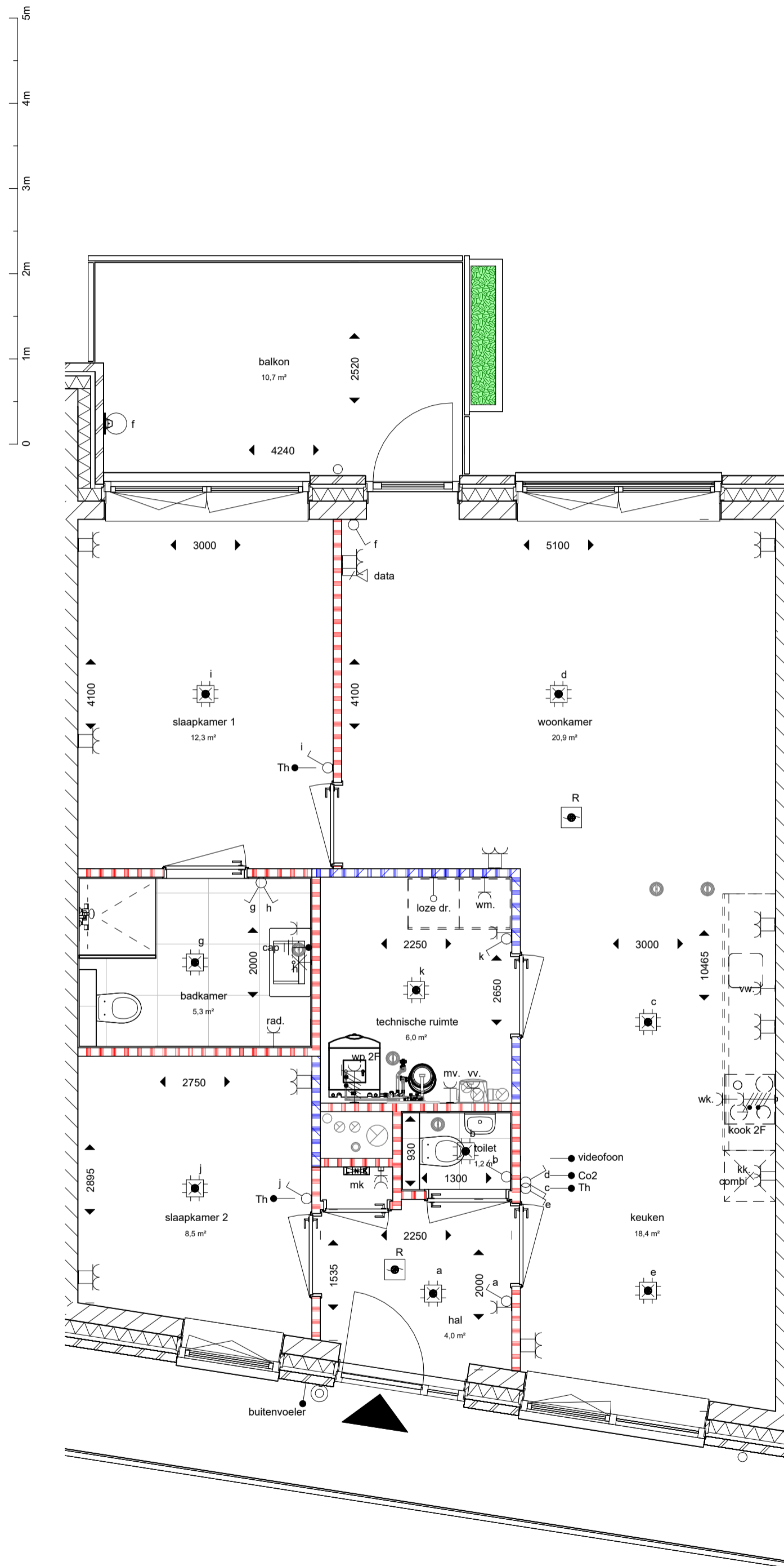
bnr 08 - type (Hyde Park) 1 : 50
