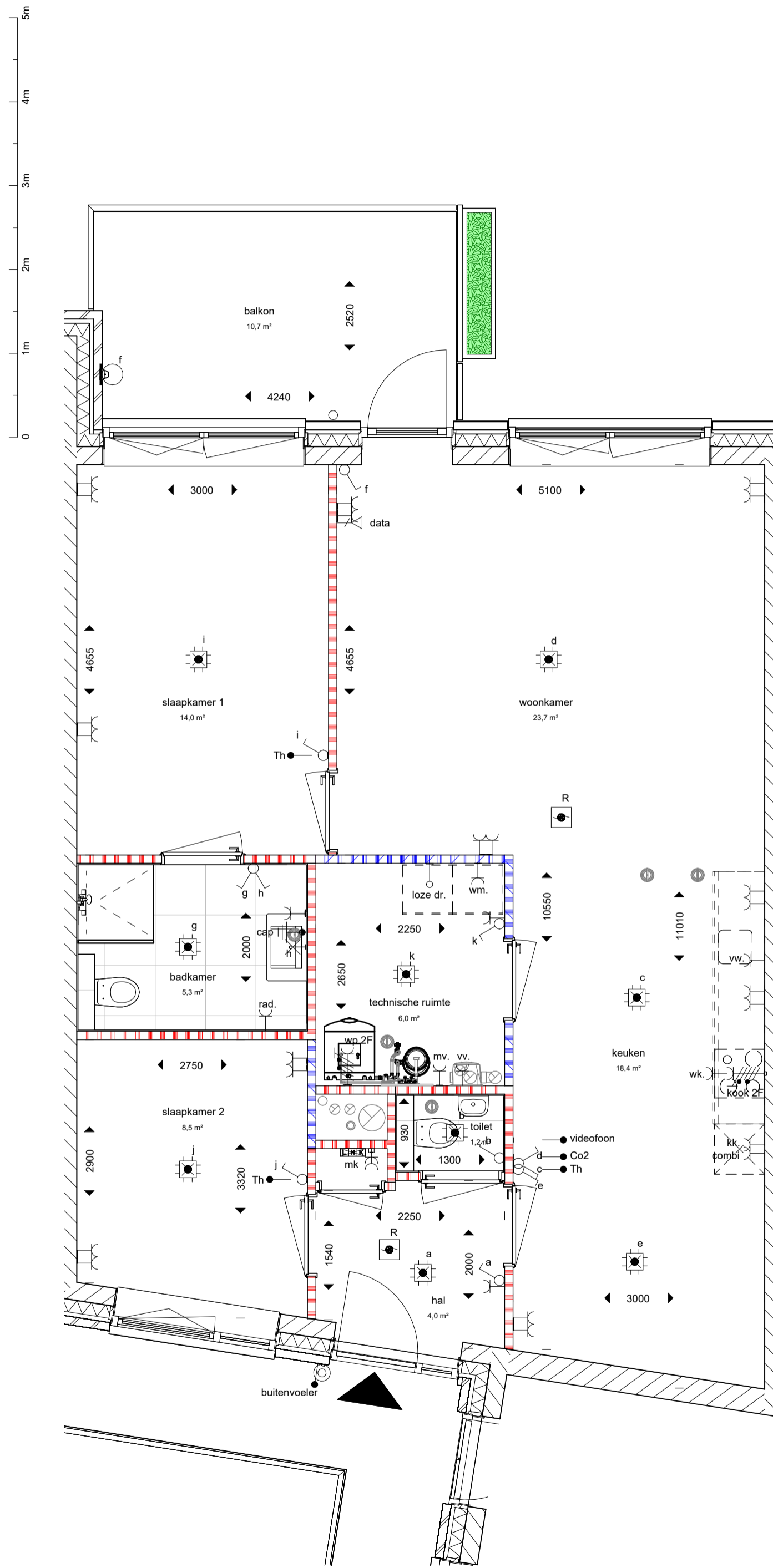
bnr 19 - type (Central Park)
