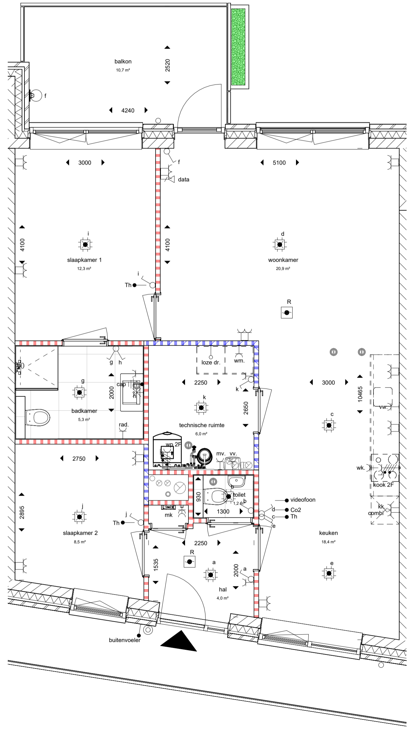
bnr 17 - type (Hyde Park) 1 : 50
