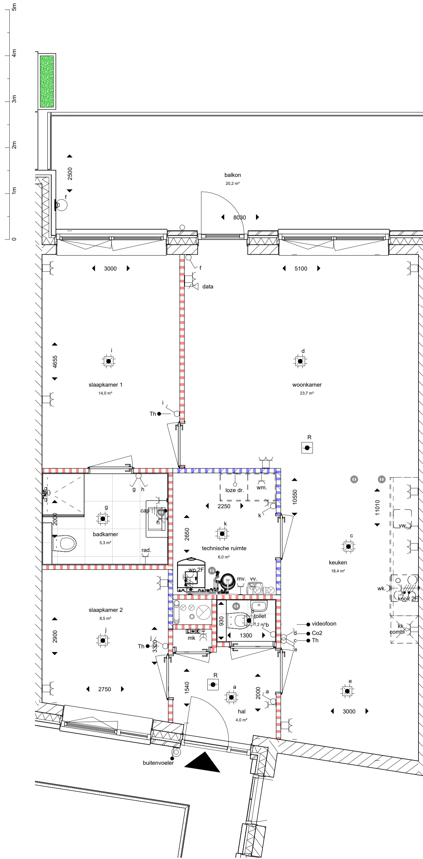
bnr 11 - type (Central Park) 1 : 50
