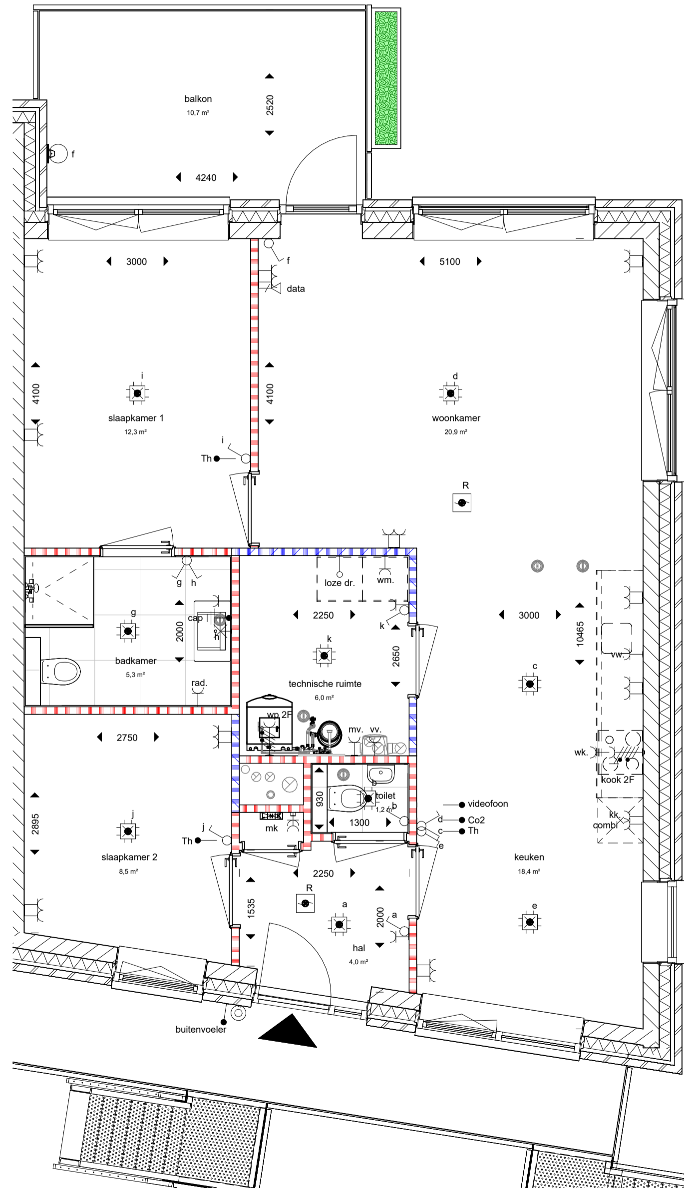
bnr 06 - type (Hyde Park) 1 : 50
