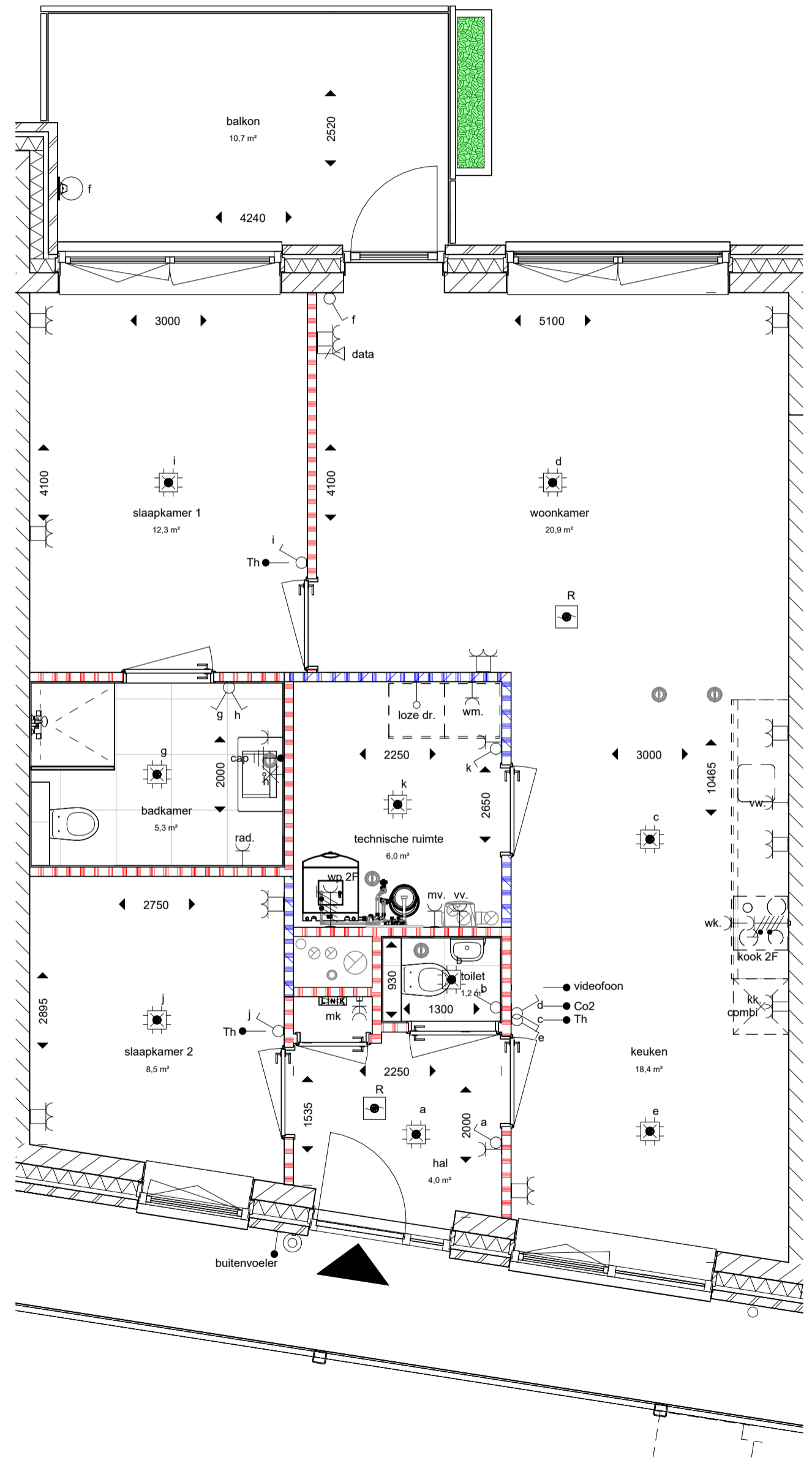
bnr 16 - type (Hyde Park) 1 : 50
